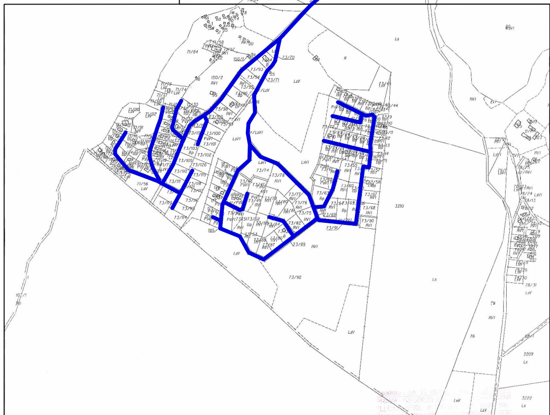
Załącznik graficzny 4.2 Sieci wodociągowe istniejące i projektowane Zasilane w wodę z SUW Sulęczyńskie
